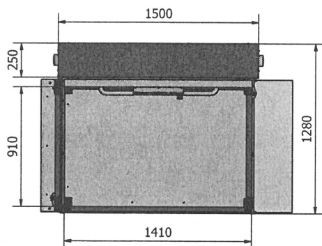
Wersja przelotowa 180°
